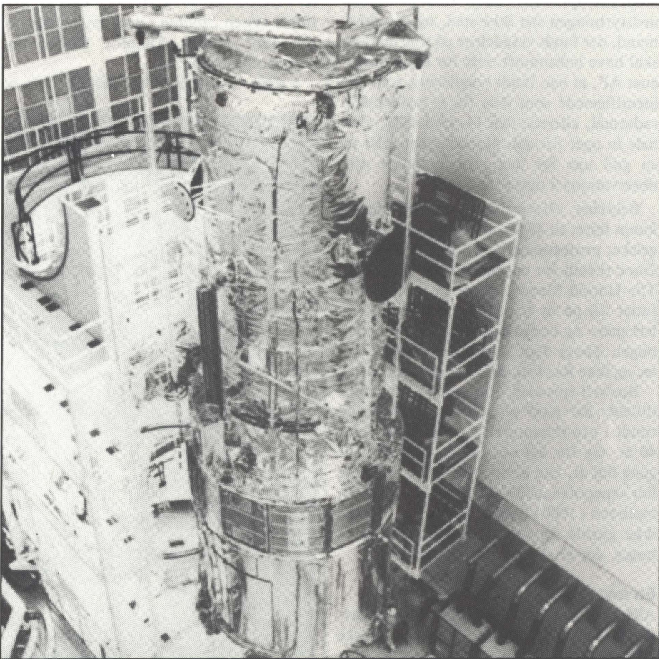
Hubble-rumteleskopet under opbygning. Teleskopet har en længde på 13,1 m, en diameter på 4,25 m og vejer i alt 11,25 tons. Man får et indtryk af den enorme størrelse ved at prøve at få øje på den medarbejder, der står forinden til højre for teleskopet.
